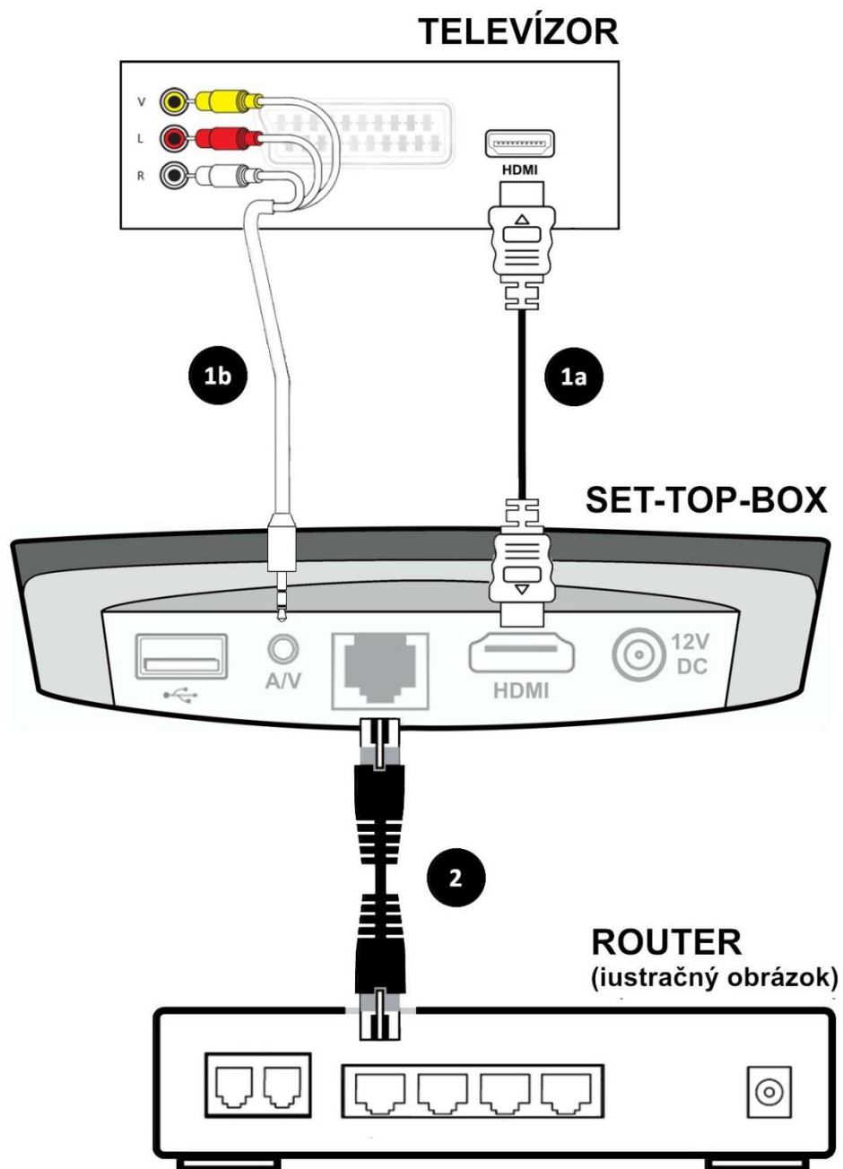
Obr. 2: Schematické znázornenie celkového zapojenia
